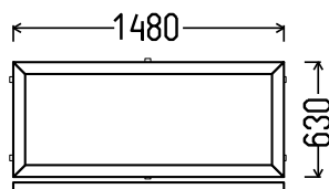
Vaizdas iš vidaus V14 (1vnt)
