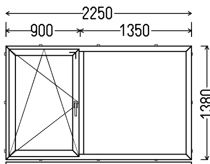
Vaizdas iš vidaus L13 (1vnt)
